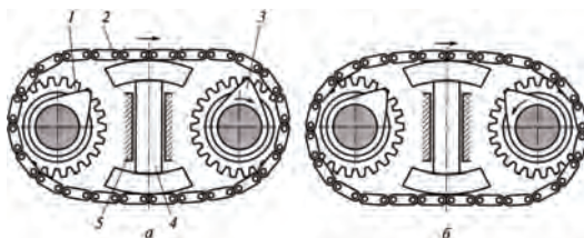
Рисунок 1. Принципиальные схемы гидромеханического устройства непрерывного регулирования фаз газораспределения впускных клапанов при максимальном (а) и минимальном (б) перекрытии клапанов.
