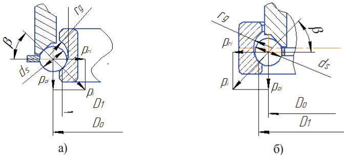
Рисунок 2 – Геометрия зоны контакта тел и дорожки качения: а) внутреннего кольца; б) наружного кольца
