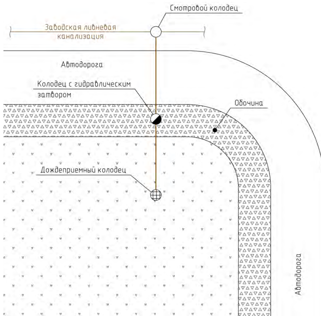
Рисунок 1 – Схема отведения поверхностных сточных вод в ливневую заводскую сеть
