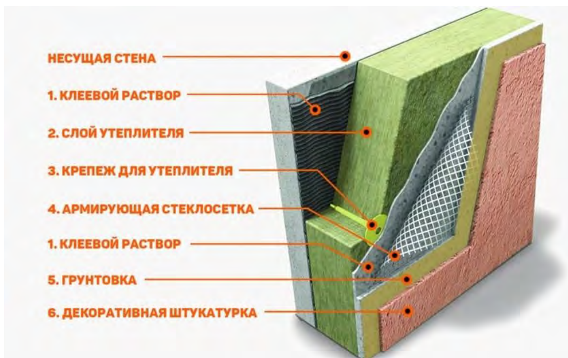
Рисунок 1 – Разрез наружной несущей стены
