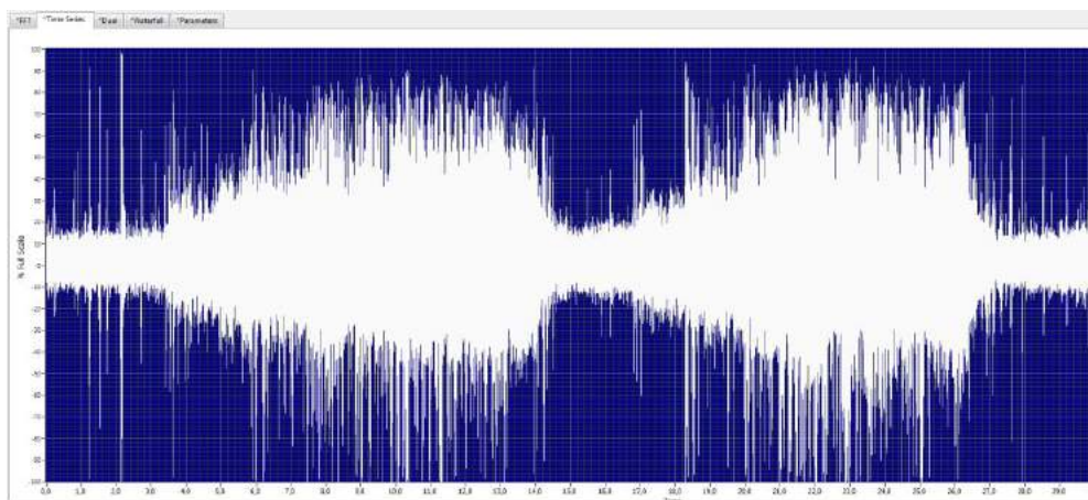
Рисунок 3 – Работа исправного конденсатоотводчика постоянного расхода
