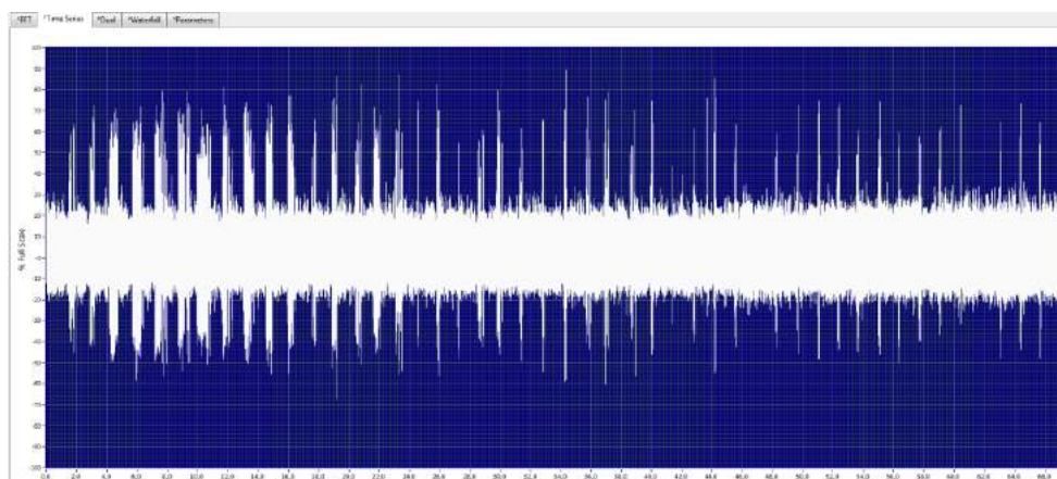
Рисунок 2 – Работа исправного конденсатоотводчика переменного расхода
